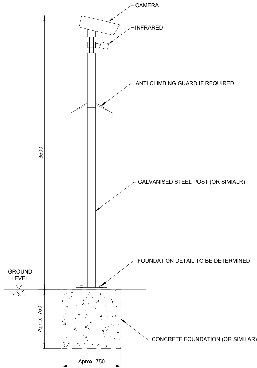
ELEVATION
